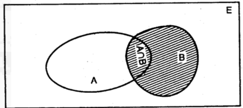
Fig. 4.7 P(A|B) .
