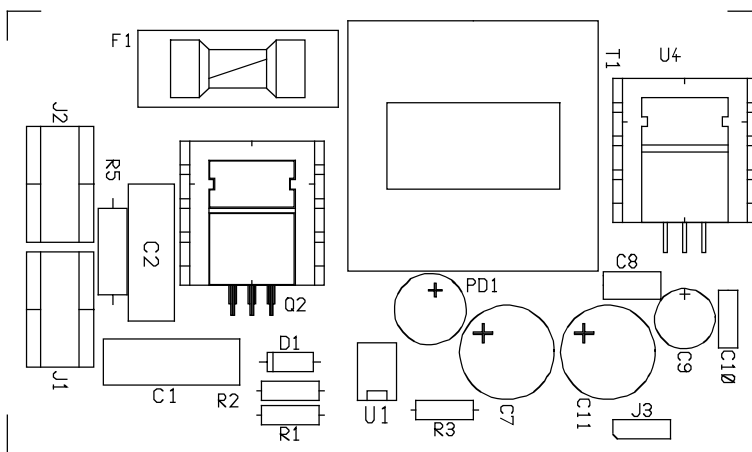
PIANO MONTAGGIO DEI COMPONENTI
