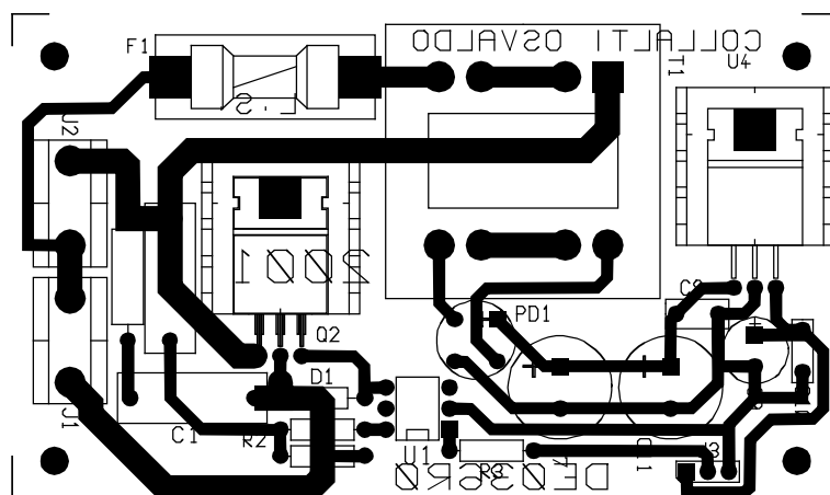
VISTA COMPONENTI E PISTE
