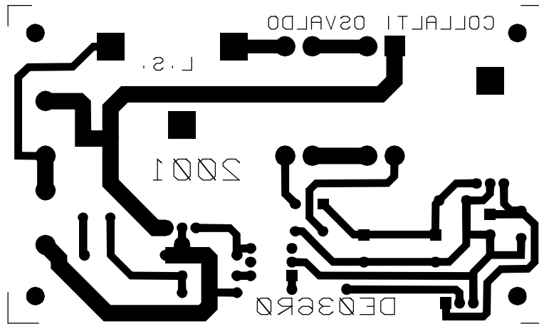
VISTA PISTE DAL LATO COMPONENTI
